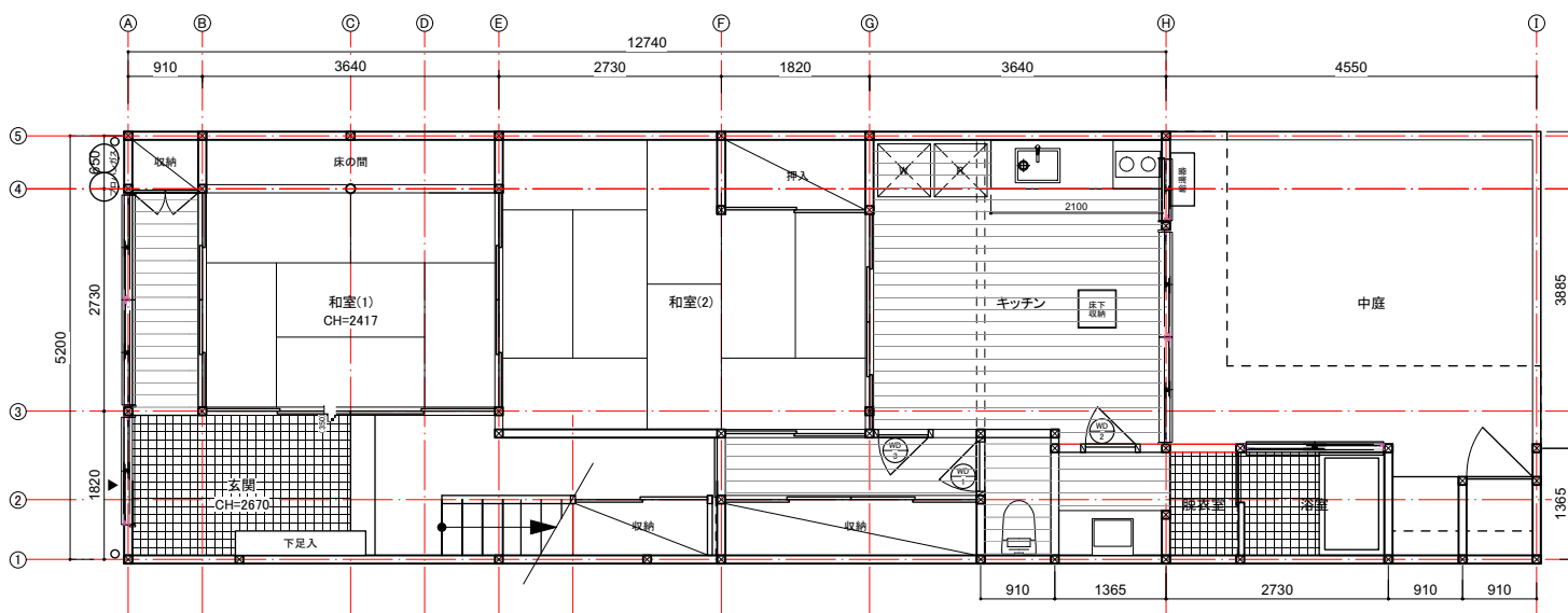
1階平面図 S=1:100 約75.77㎡
