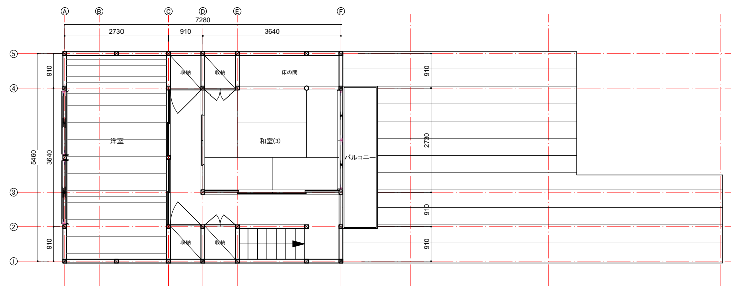
2階平面図 S=1:100 約39.74㎡
